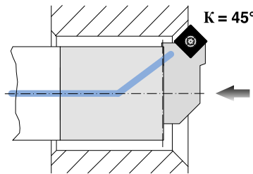
Anfasen Front- und Rückseite Front and reverse side chamfering Chanfreinage frontal et sur partie arrière
